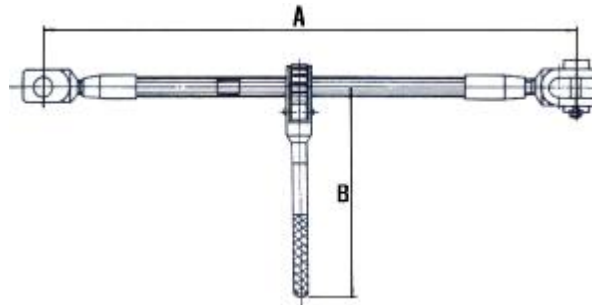
CLEVIS TYPE
